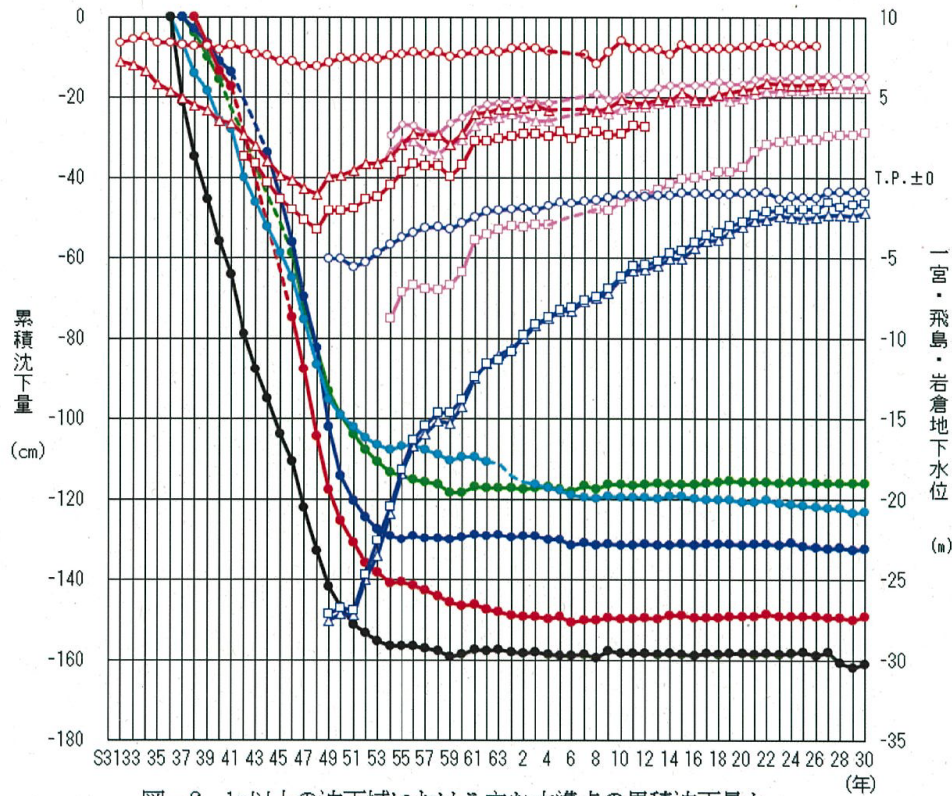
図-6 1m以上の沈下域における主な水準点の累積沈下量と 地下水位観測所の年平均地下水位の経年変化
